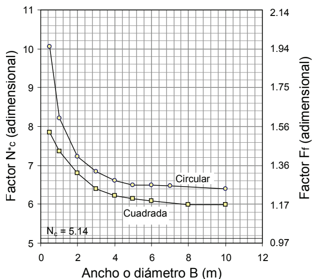
Figura 7. Factores N_c^* y F_f de losas de cimentación circulares y cuadradas desplantadas superficialmente en suelo puramente cohesivo
