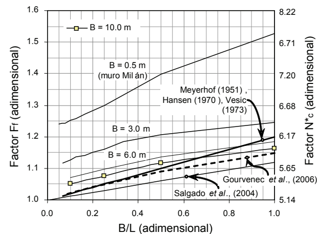
Figura 8. Factores N_c^* y F_f de losas de cimentación rectangulares desplantadas superficialmente en suelo puramente cohesivo
