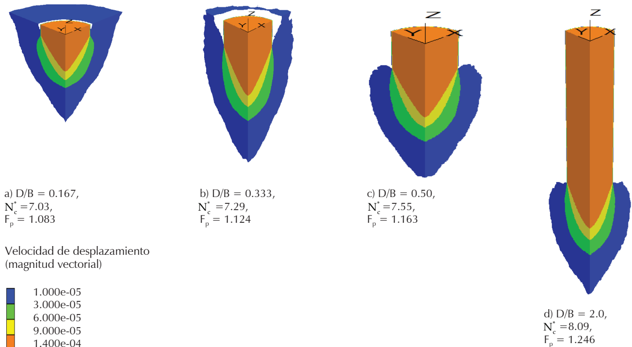
Figura 9. Contornos de velocidad de desplazamiento que definen la superficie de falla plástica de celdas circulares de diámetro B=6.0 m, vista de la cuarta parte de cada modelo
